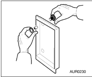
5 - Fastgør holderen
